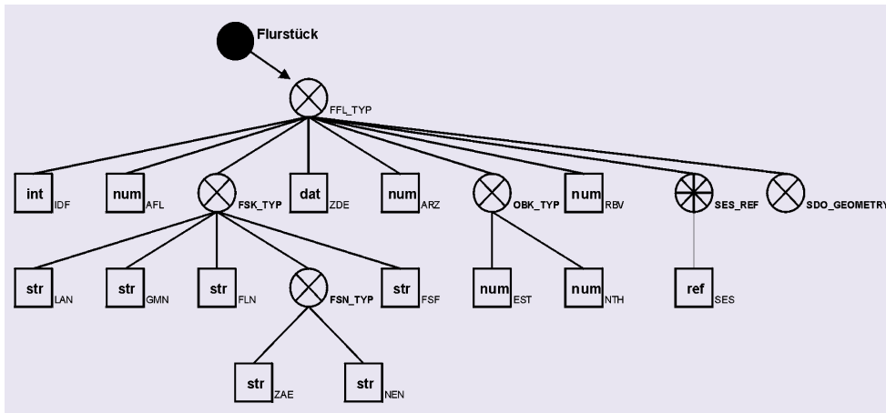
Abb. 4: Darstellung der Objektklasse Flurstück (FFL)
