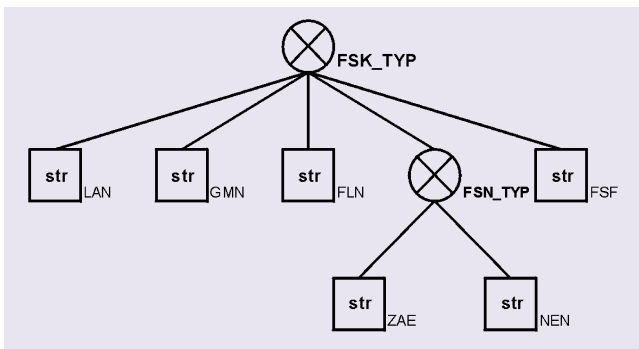
Abb. 3: Strukturierung des Attributs Flurstückskennzeichen (FSK)
