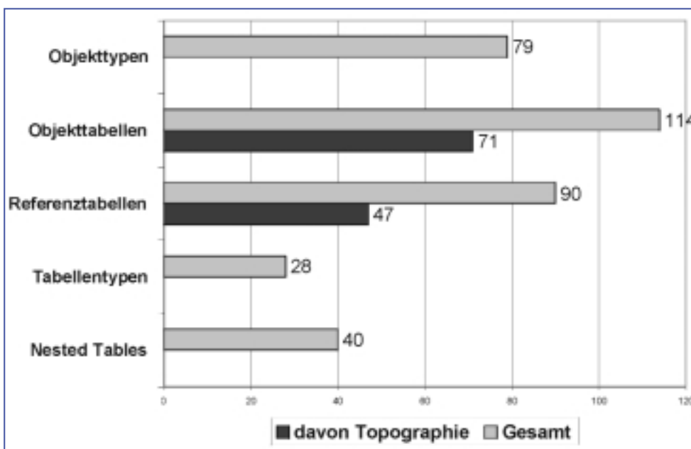
Abb. 5: Erzeugte Objekte im Datenbankschema des ALKIS®-OO-Modells
