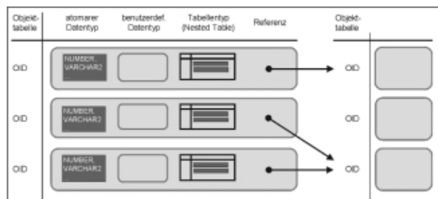
Abb. 1: Mögliche Datentypen in einer Objekttafel
