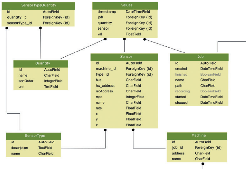
Fig. 3 | Database Schema
