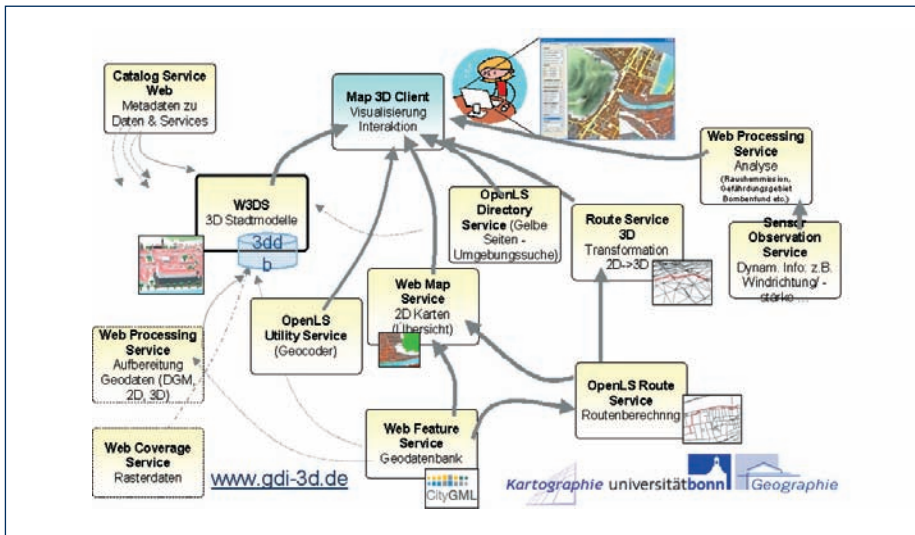
Architektur der 3D-Geodateninfrastruktur. Durch die Kombination der OGC Dienste lassen sich komplexe Anwendungen realisieren.
