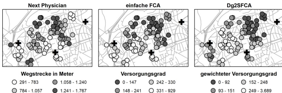
Abb. 2: Vergleich der Ergebnisse für die Augenärzte (+) in einer ausgewählten Region
