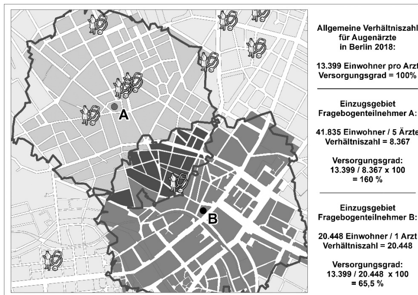
Abb. 1: Berechnung des FCA-Indikators am Bsp. der Augenärzte in Berlin
